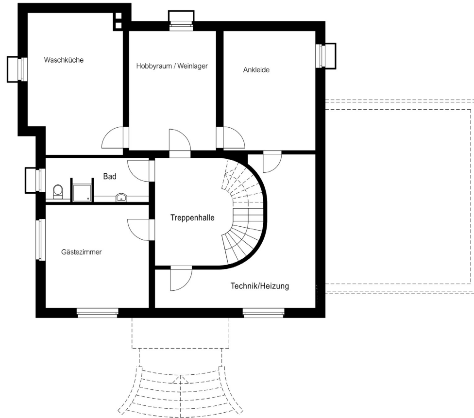
Kellergeschoss
